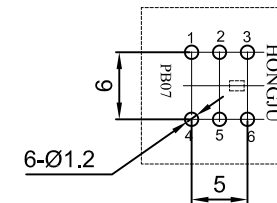
PCB HOLE( BOTTOM VIEW)
