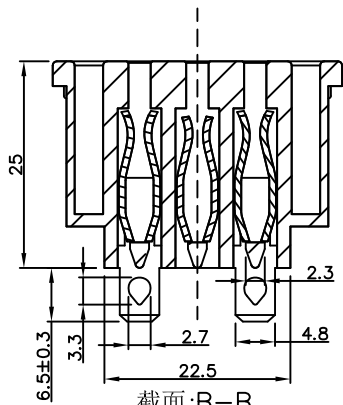
截面:B-B
